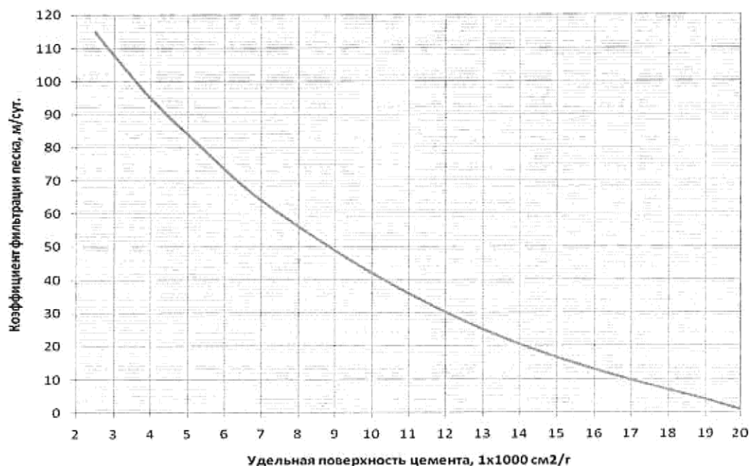
Рисунок Т.1 - График зависимости проникающей способности цементного раствора от удельной поверхности цемента и K_{\phi}
