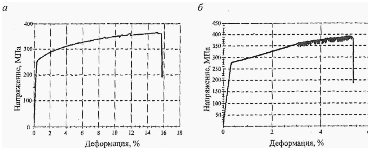
а - алюминиевый деформируемый сплав марки 1915т по ГОСТ 4784 ; б - алюминиево-магниевый сплав марки 1565ч по ГОСТ 4784
