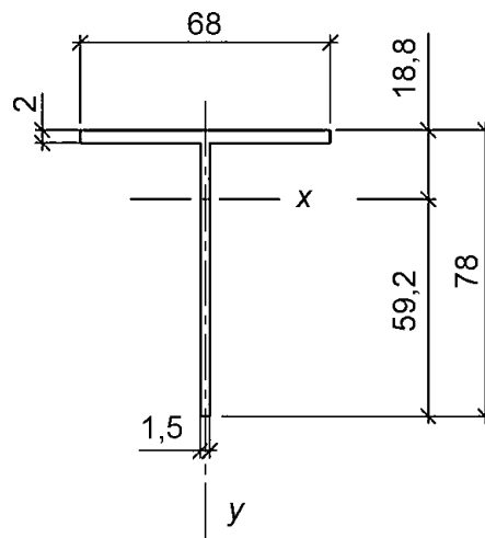
Рисунок Б.1 - Расчетное сечение направляющей
