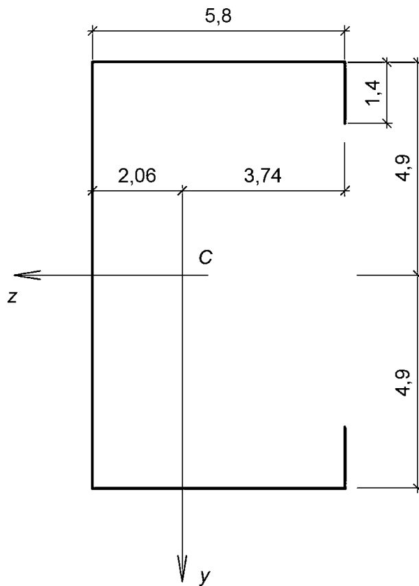
Рисунок А.3 - Расчетная схема сечения, см
