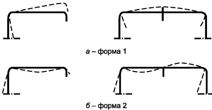
Рисунок 5 - Формы потери устойчивости подкрепленных плоских элементов
