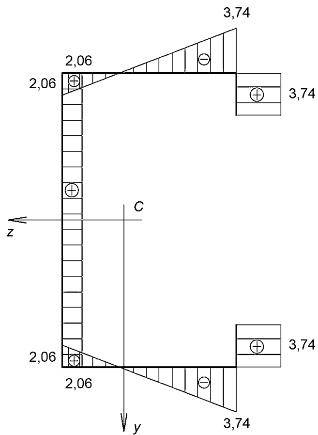
Рисунок А.4 - Эпюра координат z , см
