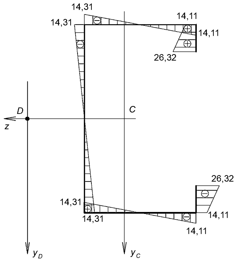
Рисунок А.9 - Эпюры главных секториальных координат
