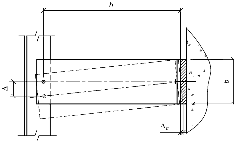
Рисунок 2 - Схема деформации прокладки под пятой кронштейна
