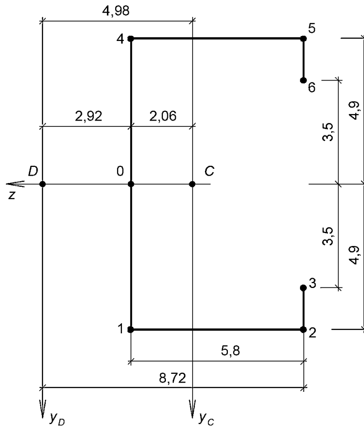
Рисунок А.8 - Положение центра изгиба
