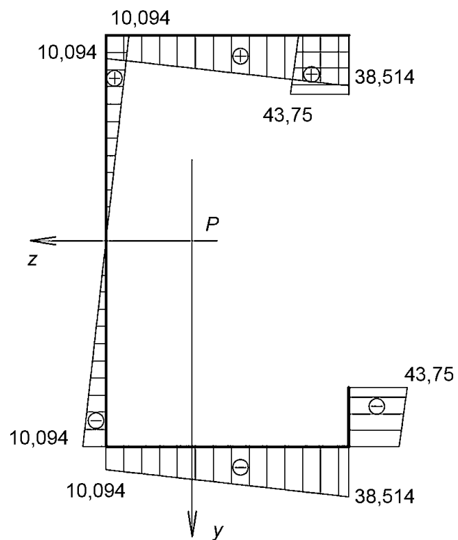
Рисунок А.6 - Эпюра секториальных координат \omega_c , см 2
