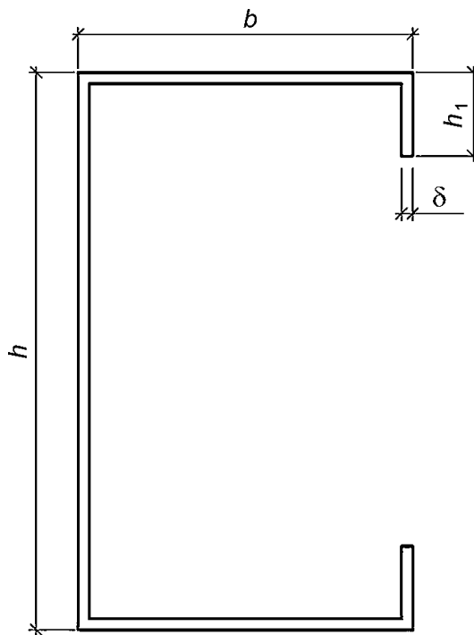
Рисунок А.1 - Схема заданного сечения
