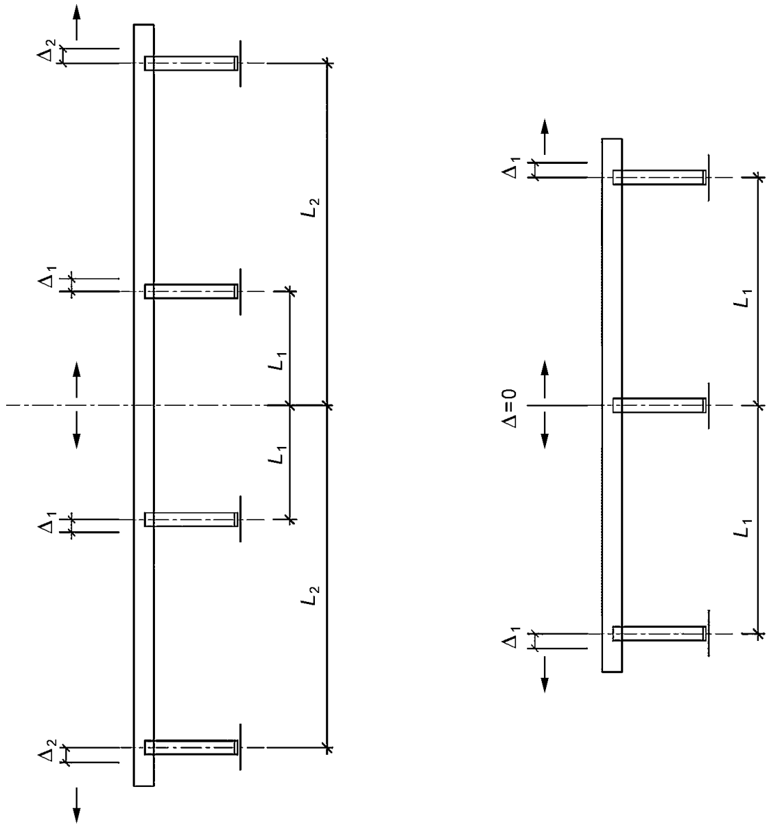
Рисунок 1 - Температурные деформации направляющей НФС
