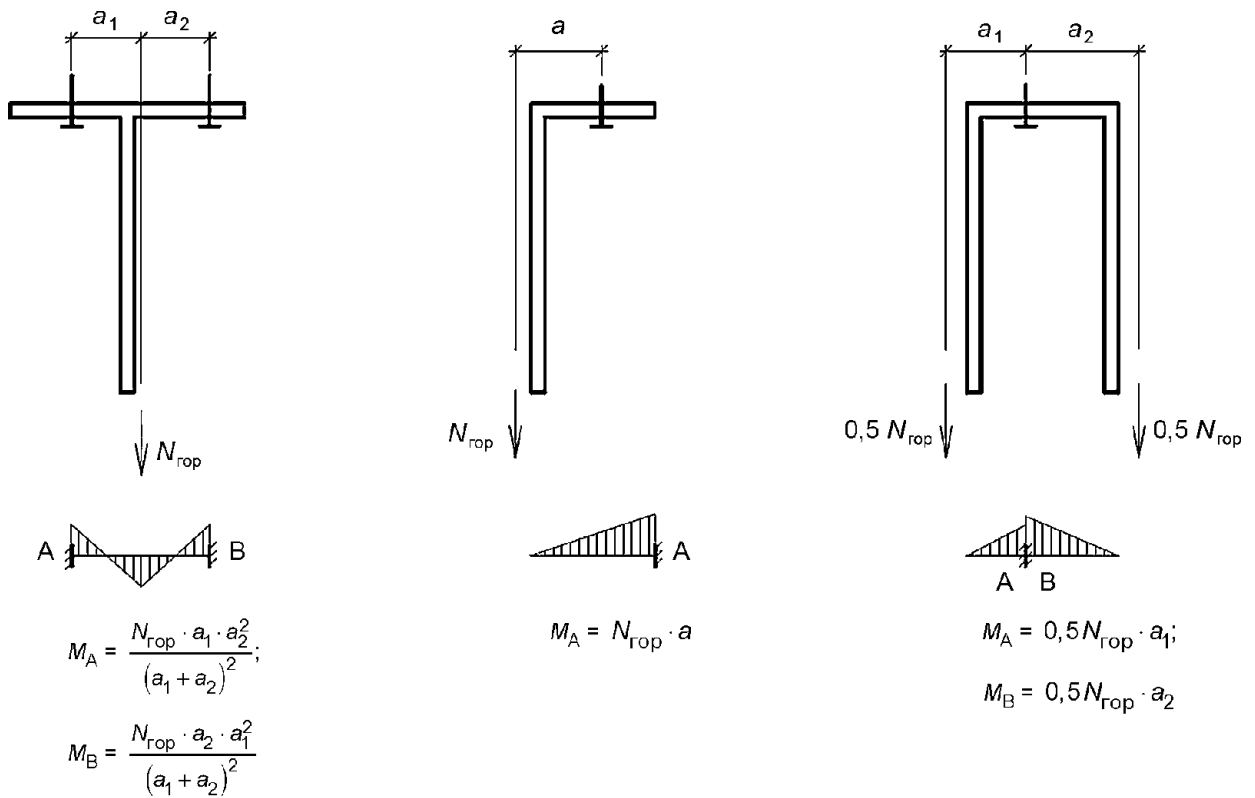
Рисунок Г.1 - Определение моментов от горизонтальной нагрузки при расчете пяты кронштейна на отгиб
