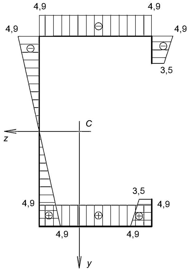
Рисунок А.5 - Эпюра координат y , см
