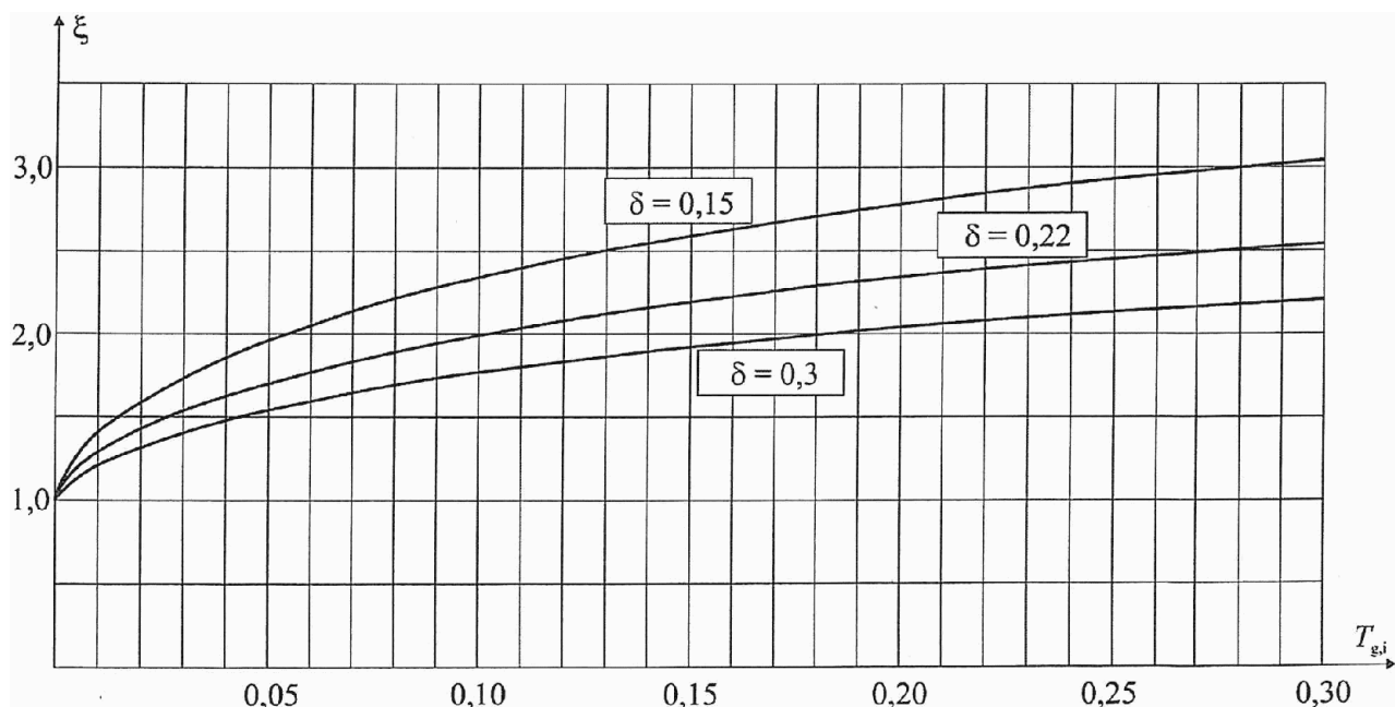
Рисунок 11.1 - Коэффициенты динамичности
