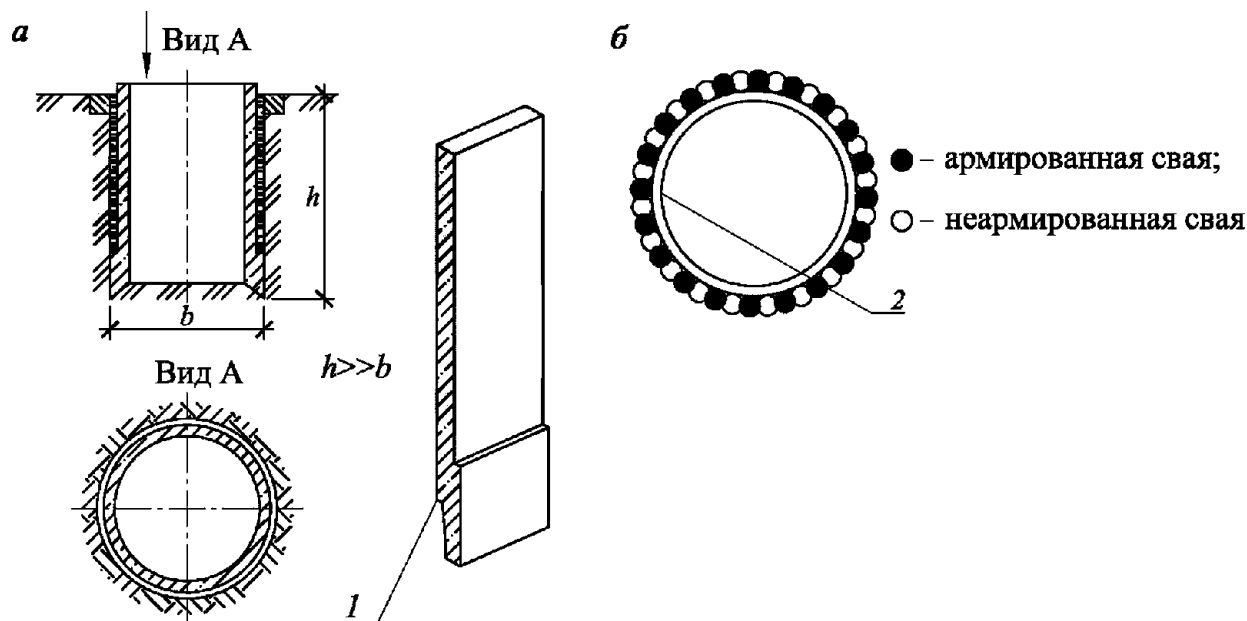
а - колодец (камера) из сборных железобетонных элементов; б - колодец (камера) из буросекущихся свай; 1 - сборный железобетонный элемент; 2 - обвязочный пояс; b - диаметр колодца (камеры); h - высота колодца (камеры), при этом h значительно больше b
