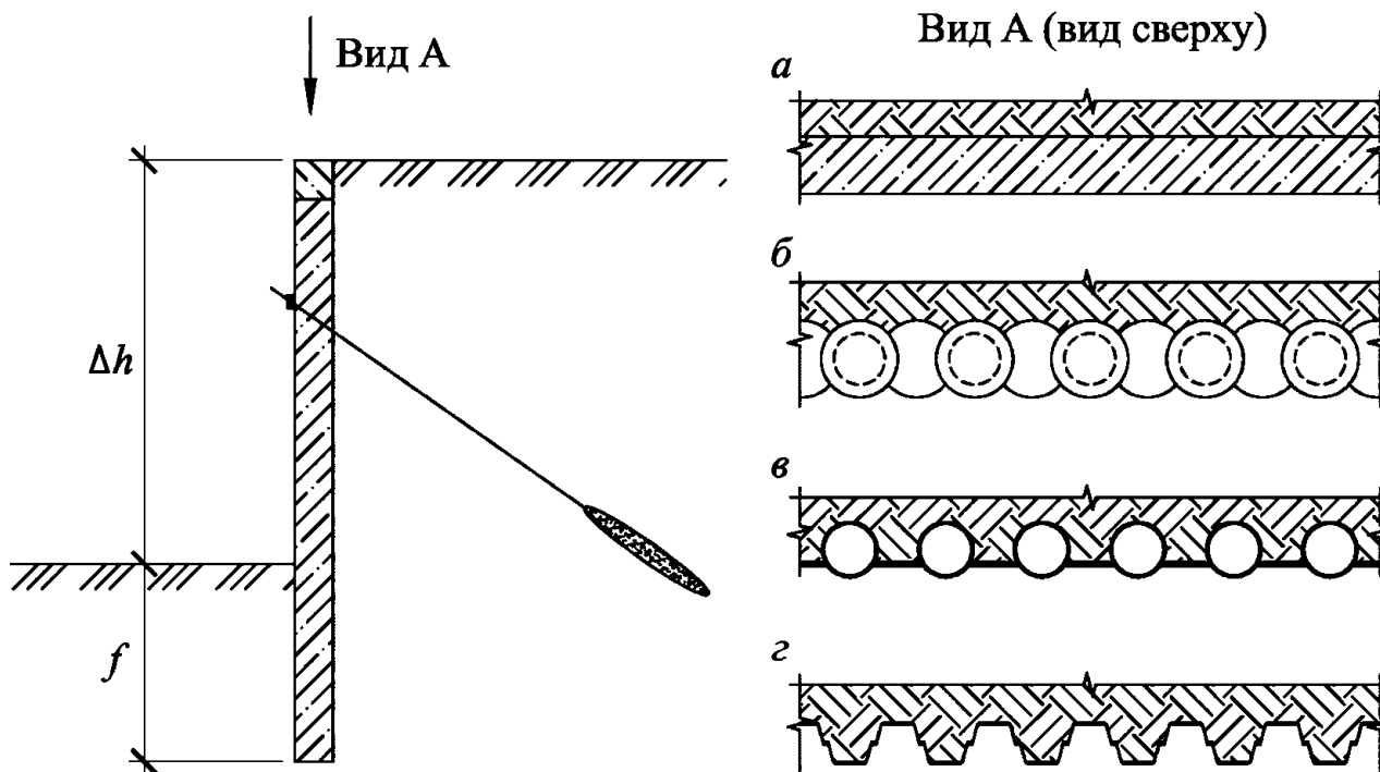
а - траншейная железобетонная "стена в грунте"; б - ограждение из буросекующихся свай; в - ограждение из металлических труб с забиркой; г - шпунтовое ограждение типа "Ларсен"; \Delta h - перепад высот; f - зона заделки
