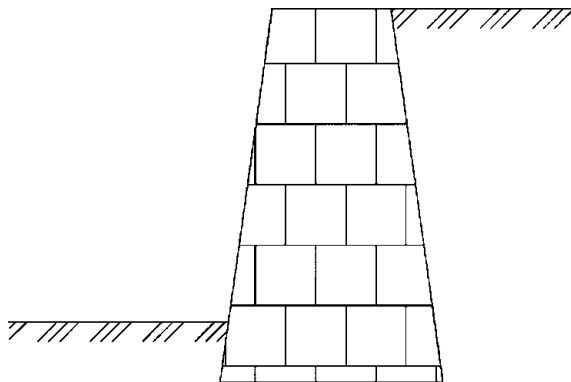
Рисунок Г.1 - Массивная подпорная стена
