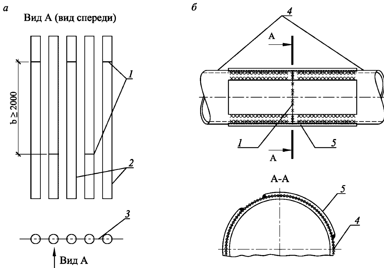
а - расположение стыков по высоте элементов по периметру сооружения; б - пример стыка металлического элемента; 1 - стыки элементов; 2 - стальные элементы подпорного сооружения; 3 - ось подпорного сооружения; 4 - стыкуемые элементы; 5 - пластины стыка
