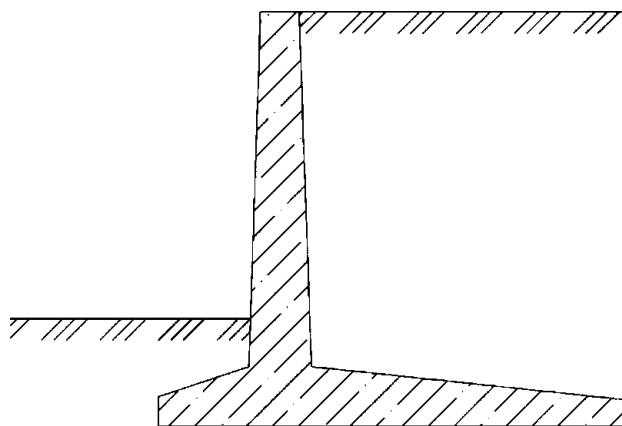
Рисунок Г.2 - Угловая подпорная стена
