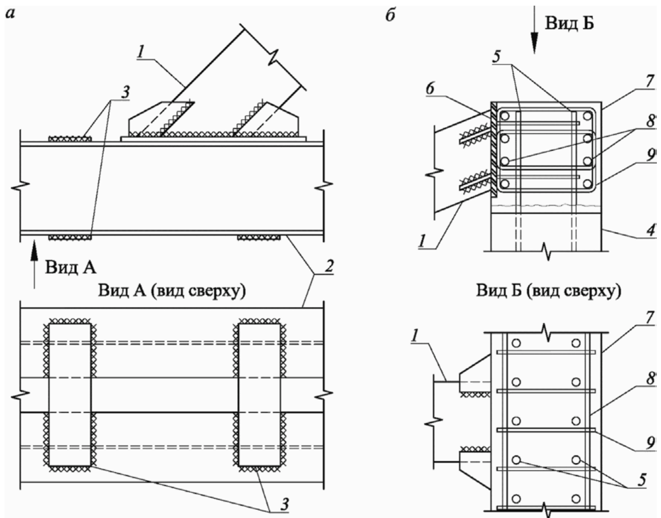
а - стального; б - монолитного железобетонного; 1 - распорка; 2 - распределительный пояс; 3 - пластины раскрепления пояса по длине; 4 - контур подпорной стены; 5 - армирование подпорной стены; 6 - закладная деталь; 7 - контур распределительного пояса; 8 - продольное армирование распределительного пояса; 9 - поперечное армирование распределительного пояса
