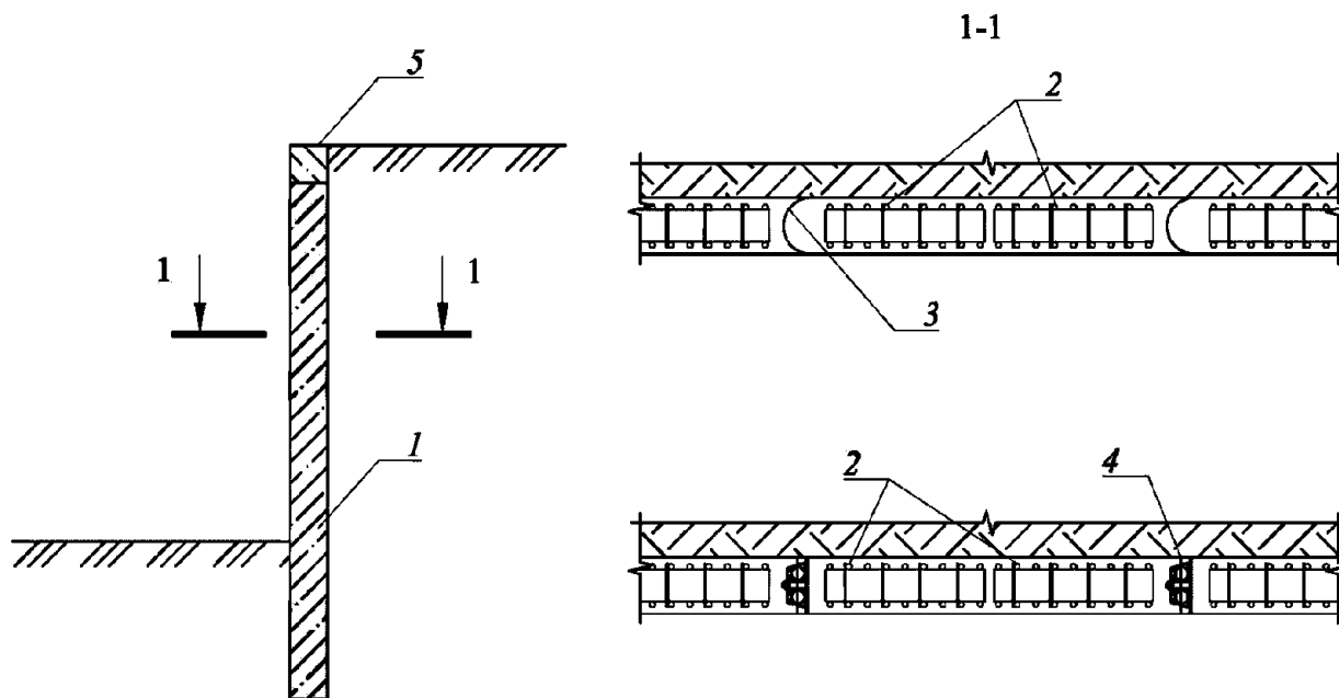
1 - "стена в грунте"; 2 - арматурный каркас; 3 - ограничитель захваток полукруглого типа;
