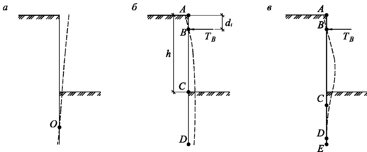
а - консольной; б - с одним ярусом крепления, метод Якоби; в - с одним ярусом крепления, метод Блюма-Ломейера
