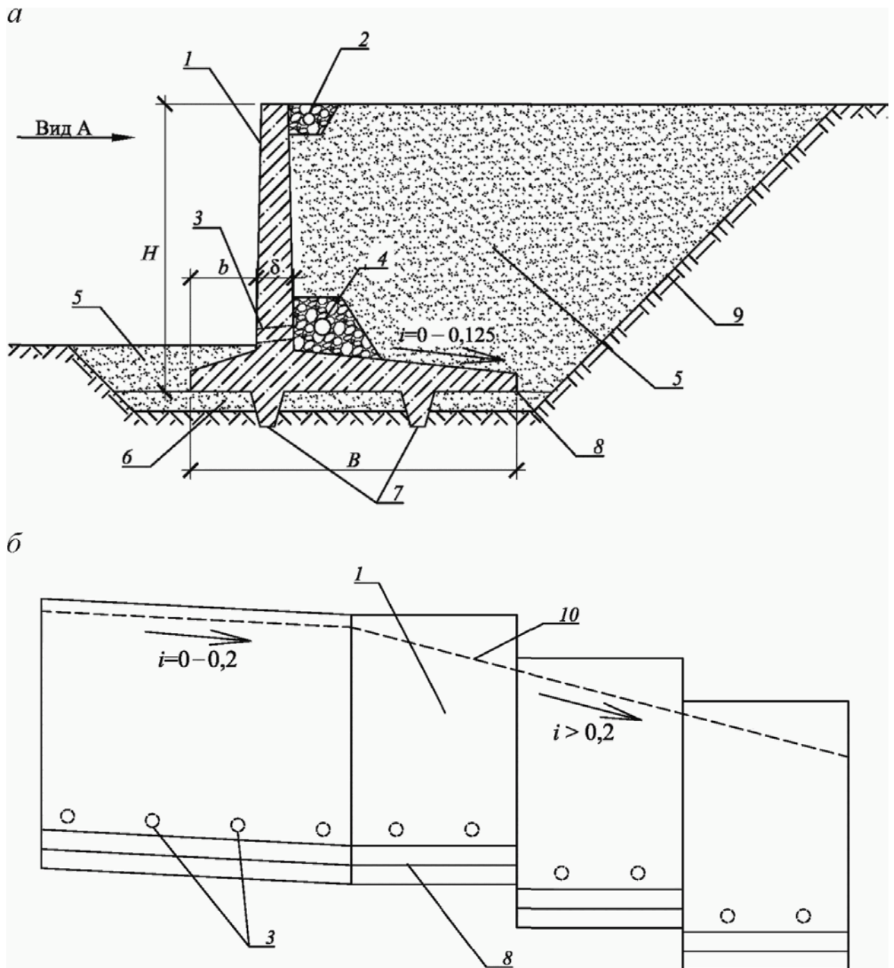
а - поперечное сечение; б - вид спереди (вид А); 1 - лицевая стенка; 2 - водоотводной кювет; 3 - дренажные трубки (шаг ~ 3 - 6 м); 4 - пристенный дренаж; 5 - обратная засыпка; 6 - подготовка основания "постель"; 7 - "зуб"; 8 - фундаментная плита; 9 - контур траншеи; 10 - контур поверхности земли; i - уклон
