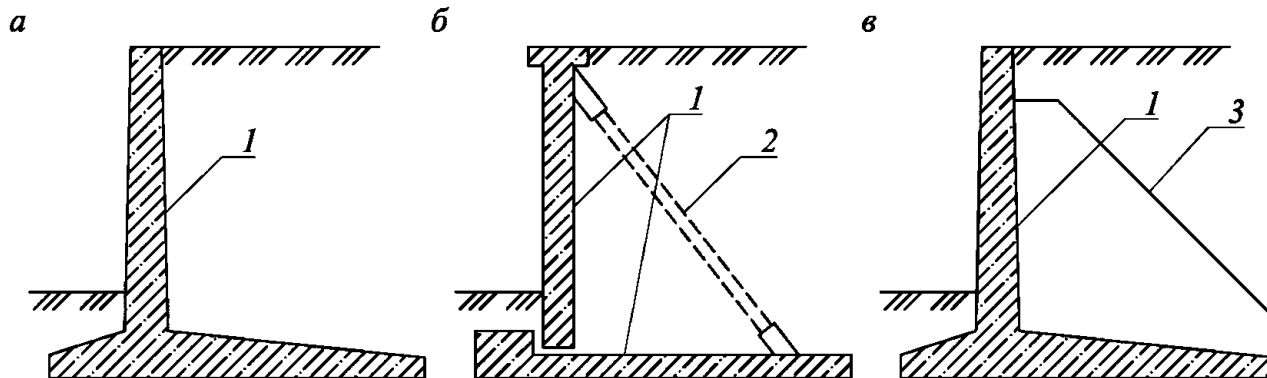
а - консольные; б - с анкерными тягами; в - контрфорсные; 1 - подпорная стена; 2 - тяга; 3 - контрфорс
