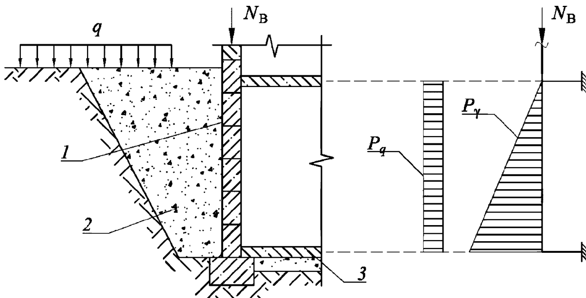
1 - стена подвала; 2 - обратная засыпка; 3 - плита пола подвала; p_q - давление от нагрузки
