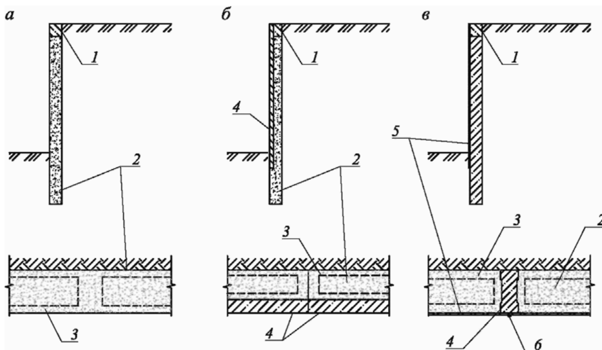
а - монолитная; б - сборно-монолитная; в - сборно-монолитная с теплоизоляцией; 1 - обвязочная балка; 2 - монолитный участок; 3 - арматурный каркас; 4 - сборная панель; 5 - теплоизоляция; 6 - сварной шов
