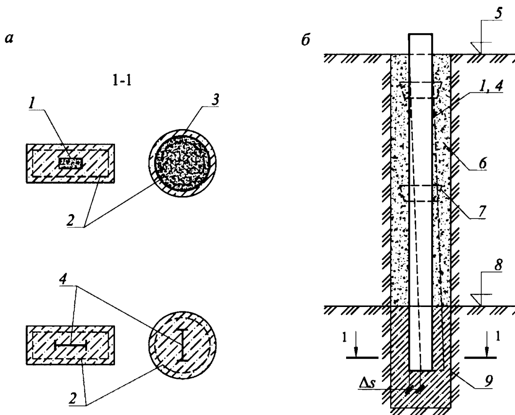
а - поперечное сечение; б - продольное сечение, отклонение от вертикали; 1 - железобетонная опора перекрытия; 2 - арматурный каркас; 3 - опора из стальной трубы с железобетонным заполнением; 4 - стальная опора перекрытия; 5 - рабочая площадка; 6 - засыпка щебнем; 7 - опорный столик; 8 - отметка разработки; 9 - фундамент опоры; \Delta s - отклонение опоры
