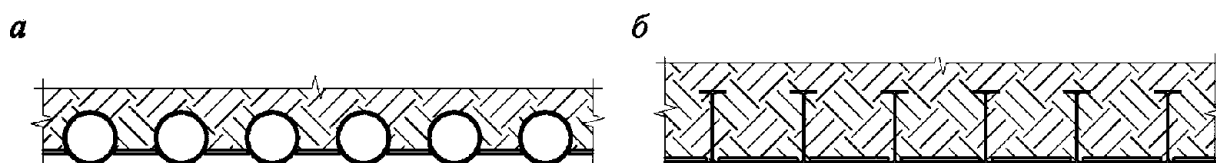
а - ограждение из металлических труб с забиркой; б - ограждение из прокатных профилей
