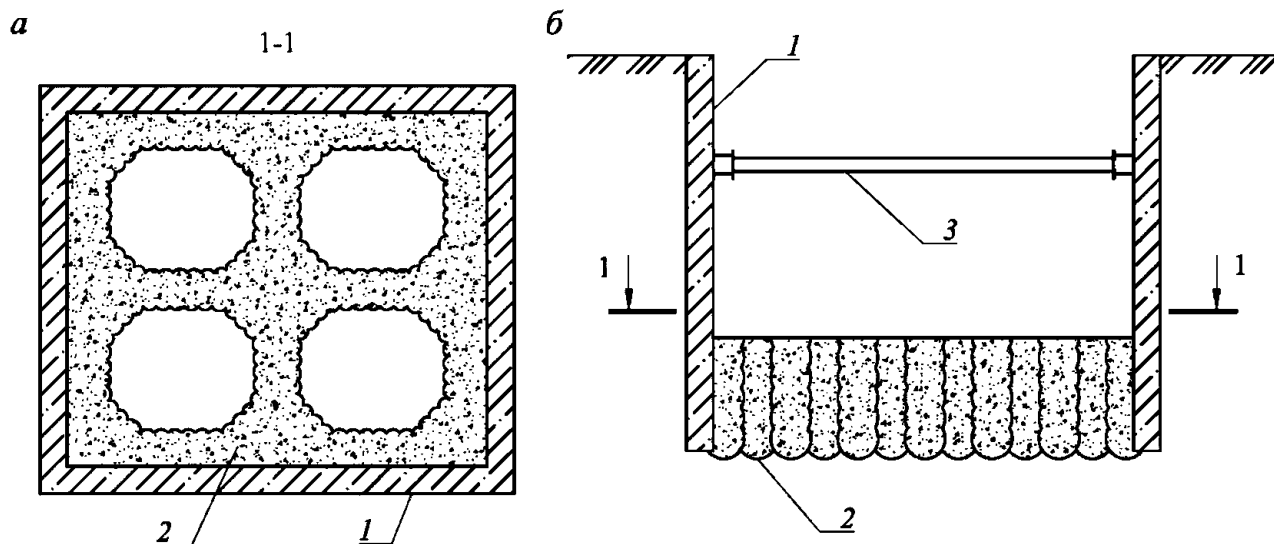
а - план; б - сечение; 1 - подпорное сооружение; 2 - укрепленный грунт заделки; 3 - распорка
