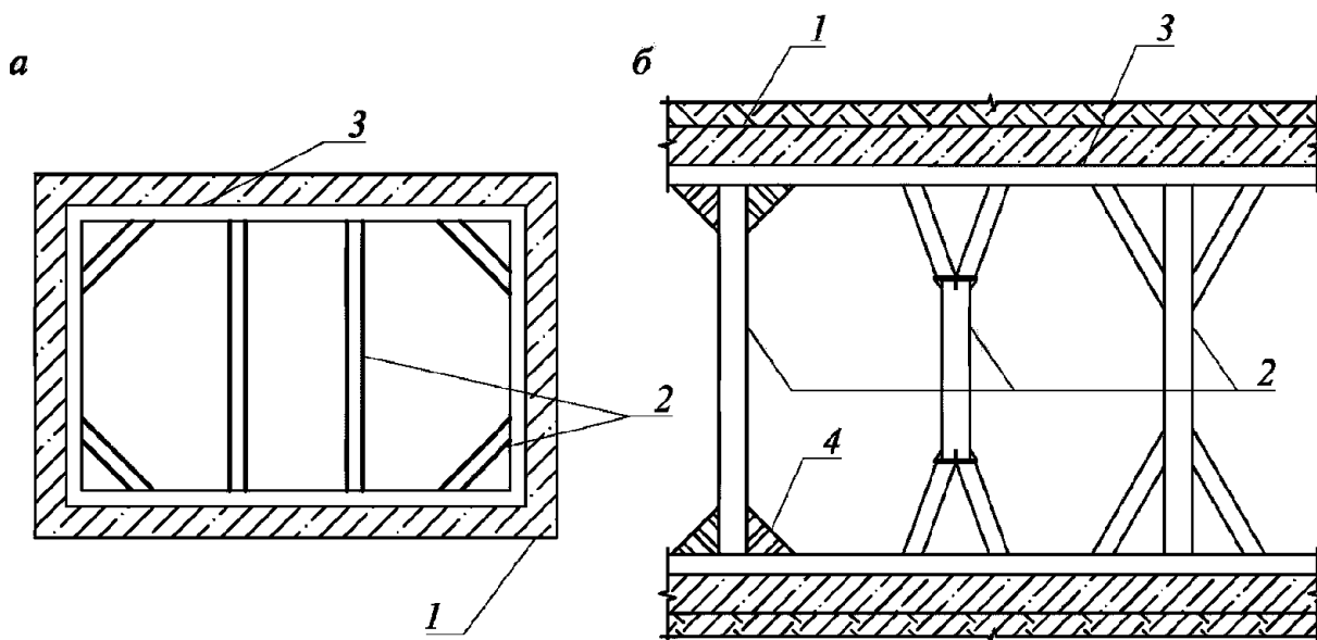
а - схема расстановки распорных элементов в плане при рядовом шаге распорок; б - примеры узлов опирания распорных элементов при большом шаге распорок в плане;
